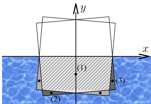
Obr. 6: Skúmanie stability polohy hranola s niektorou stranou vodorovnou. Obrázok naznačuje hľadanie polohy ponorenej časti hranola diskutované v nasledujúcom odstavci. Sivo naznačený štvorec naznačuje polohu hranola vychýlený o rovnaký uhol do opačnej strany.
