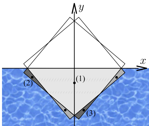
Obr. 7: Skúmanie stability polohy hranola s jednou uhlopriečkou vodorovnou. Obrázok naznačuje hľadanie polohy ponorenej časti hranola diskutované v nasledujúcom odstavci. Sivo naznačený štvorec naznačuje polohu hranola vychýlený o rovnaký uhol do opačnej strany.
