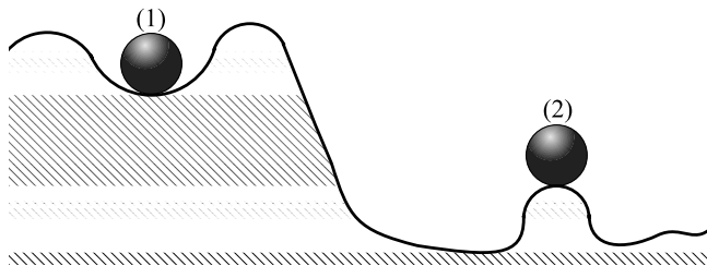
Obr. 5: Poloha (1) je stabilná a poloha (2) je labilná, hoci pre energie guľiek platí E_1 > E_2 . Očividne teda neplatí tvrdenie, že stabilná poloha je stav s najnižšou energiou. Na vznik stabilnej polohy stačí akákoľvek malá jamka.
